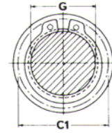
Anillo circular en ranura
